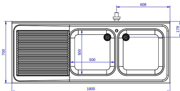
Boven aanzicht
